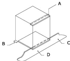
Fig. 7: Requisitos de ventilação e recorte para a instalação de um forno eléctrico simples numa unidade de cozinha standard.
